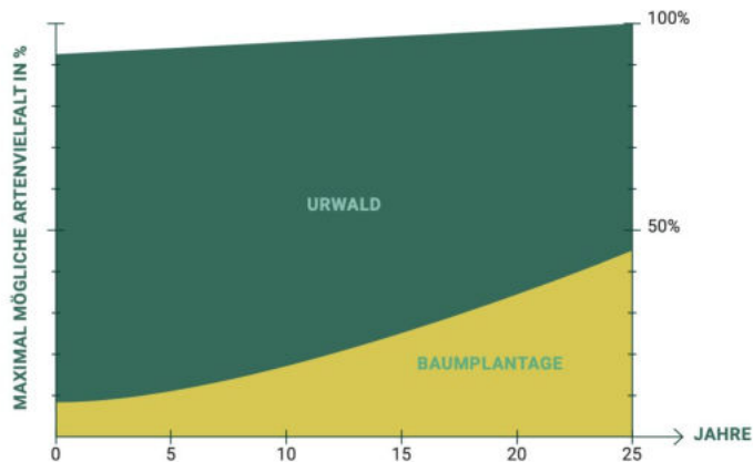
Artenvielfalt: Urwald vs. Baumplantage
