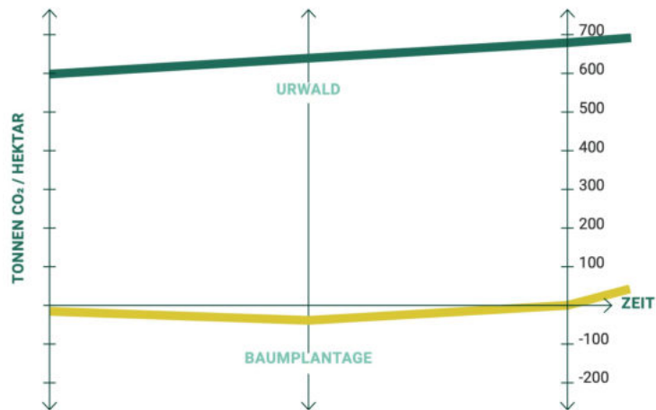
CO 2 Speicherung: Urwald vs. Baumplantage
